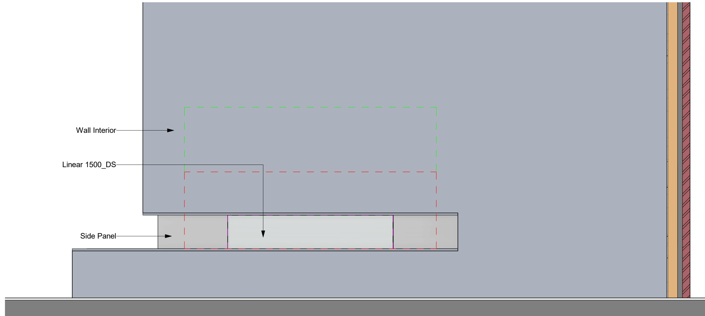
Elevation Back 1 : 20
